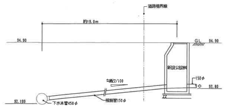
下水取付管断面図 S=1/50
